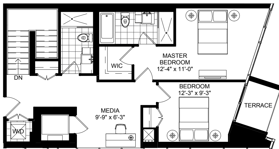
Upper
